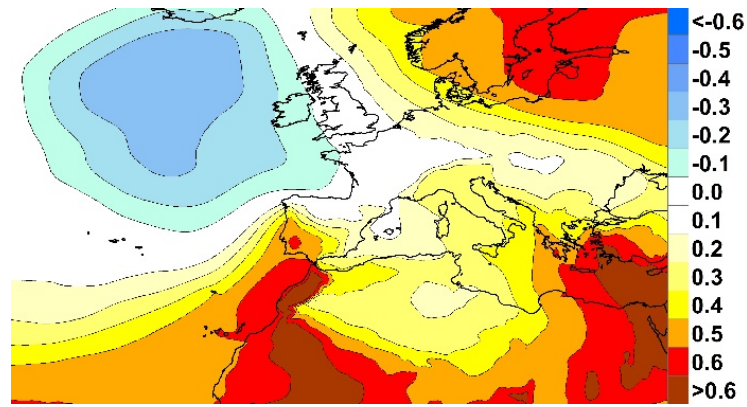
Figura 2 - Correlación presión a nivel del mar-ENSO para los meses de julio-agosto. Fuente: Sánchez-Laulhé y Núñez, 2023
