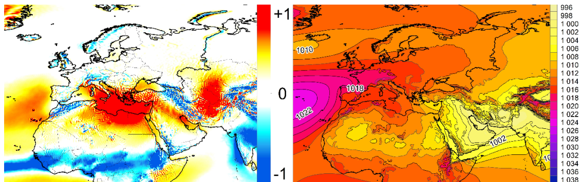
Figura 1 - Mapas climatológicos de verano (junio-agosto) de: velocidad vertical omega (en Pa/s) en 500 hPa; valores positivos descendencias (izquierda); presión a nivel del mar en hPa (derecha). Fuente ERA5
