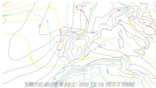
Figura 3 – Altura de geopotencial (m) en 500 hPa -líneas amarillas- ; isotermas (°C) en 850 hPa - líneas grises continuas- y en 500 hPa –líneas azules discontinuas- a las 15 UTC del 12 de julio 1935. (NOAA 20th Century Reanalysis V3)
