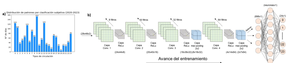
Figura 1 – a) Histograma del número de días asignados de forma subjetiva a cada patrón de la clasificación de Font durante el período 2020-2023. b) Esquema de la arquitectura de la red neuronal convolucional empleada en este trabajo.
