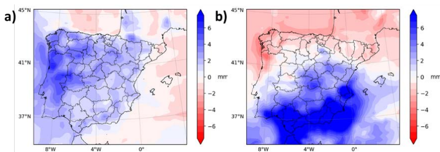
Figura 2 - Anomalías de precipitación obtenidas durante los días en los que el clasificador asignó el marco sinóptico a las situaciones de Font 12 (depresión atlántico-ibérica, a) y 13 (depresión en el golfo de Cádiz, b).
