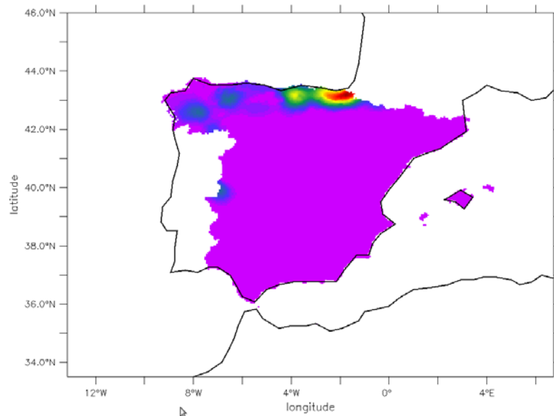
Figura 1 - Dominio de estimación. Ejemplo de precipitación acumulada diaria regionalizada para un día problema.
