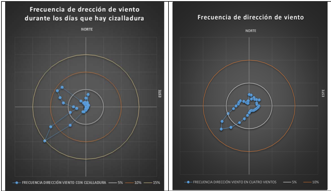
Figura 1 - Frecuencia de la dirección del viento cuando hay cizalladura (izquierda) y climatológica (derecha) durante el período 2012-2021 en el aeródromo de Cuatro Vientos.
