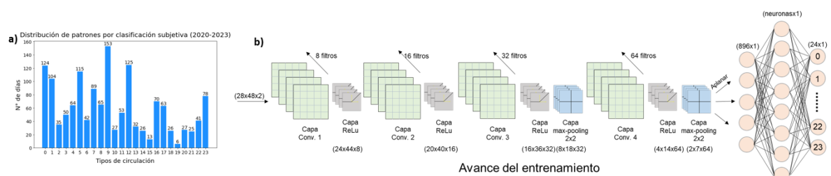
Figura 12 – a) Histograma del número de días asignados de forma subjetiva a cada patrón de la clasificación de Font durante el período 2020-2023. b) Esquema de la arquitectura de la red neuronal convolucional empleada en este trabajo.
